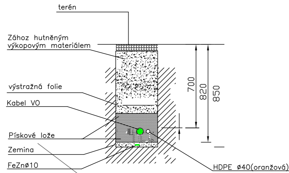
Typický řez trasou
