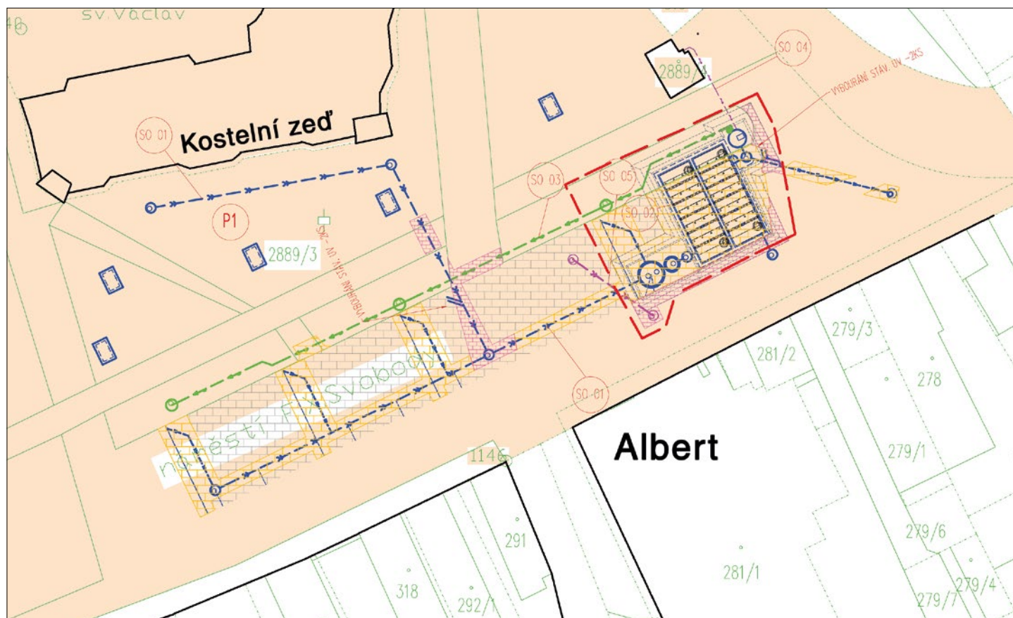
Ve výkresu je modrou linií označena nádrž a nová vedení kanalizace, zelenou nová vedení vodovodu a červenou oblast předpokládaného výkopu pro nádrž.
